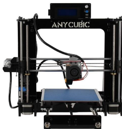
Fig: anycubic prusa i3
