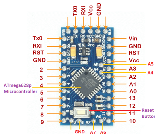
Figure 3.2: Arduino Pro Mini Pin Out
